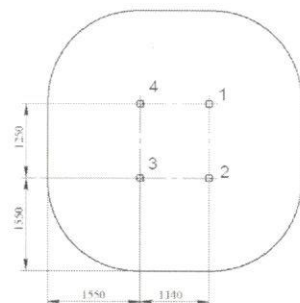
Scheme of the post placing with foundations (Схема расположения фундаментов со стойками)
